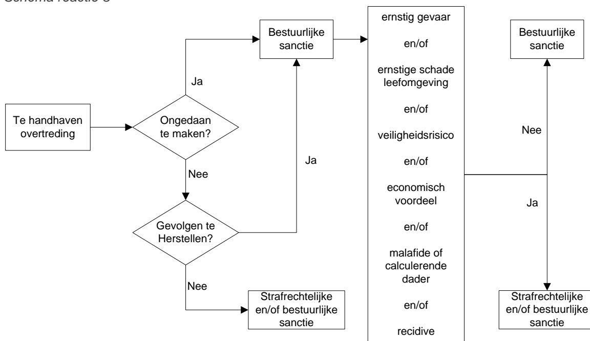
Schema reactie 3
