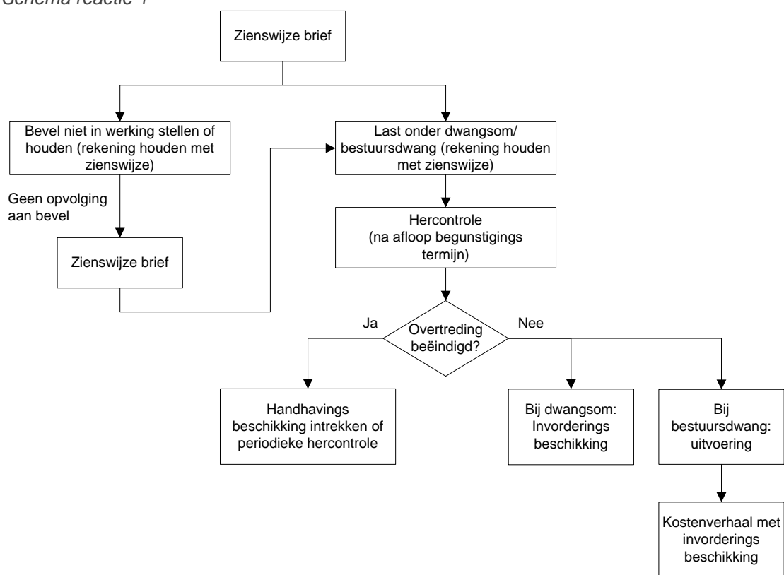
Schema reactie 1
