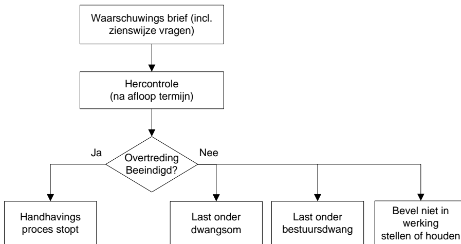
Schema reactie 2
